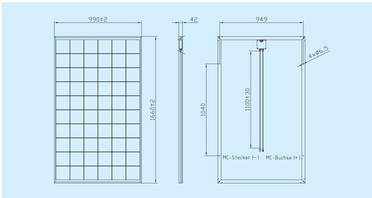
Maßzeichnung IBC-220TA MEGALINE
